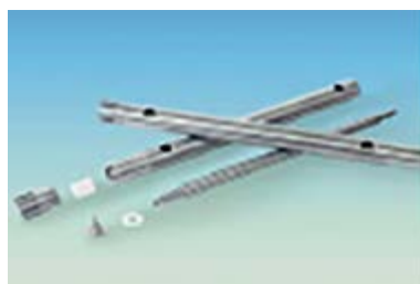
(3)(4) Насадка НТ1018
